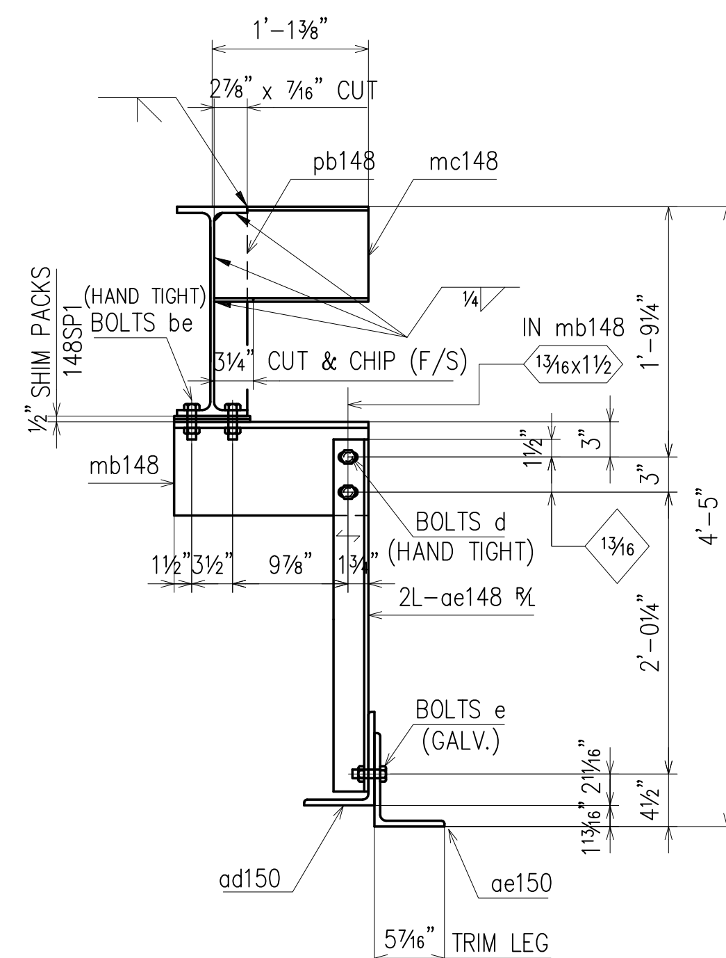
SECTION 2A
