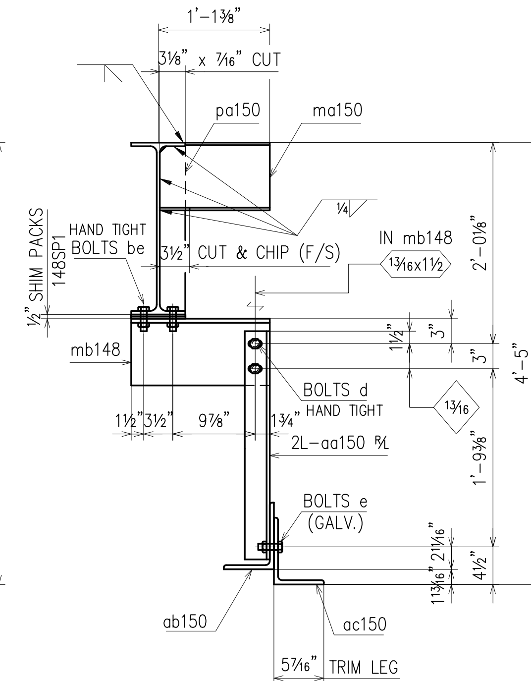
SECTION 1A
